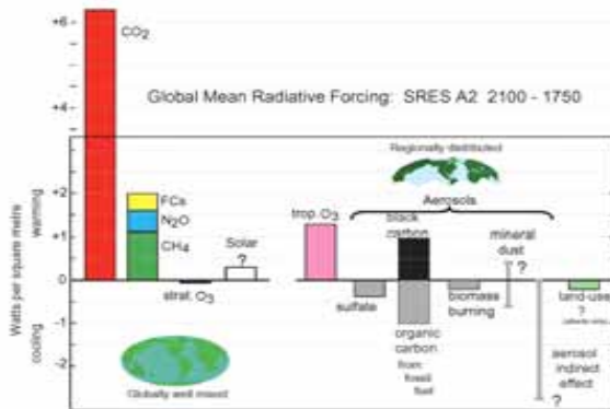
2100-1750年の全球平均放射強制力 (SRES A2)
