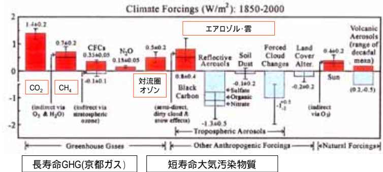
各地球温暖化関連物質による1850-2000年の放射強制力
