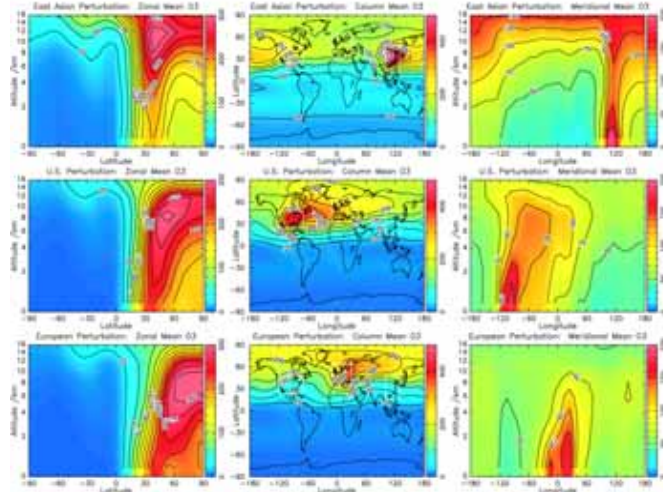
O. Wild, H. Akimoto, J. Geophys. Res., 106, 27,729 (2001)
