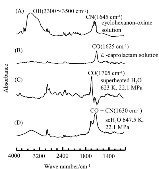
図1 超臨界水ベックマン転位反応のIRスペクトル
