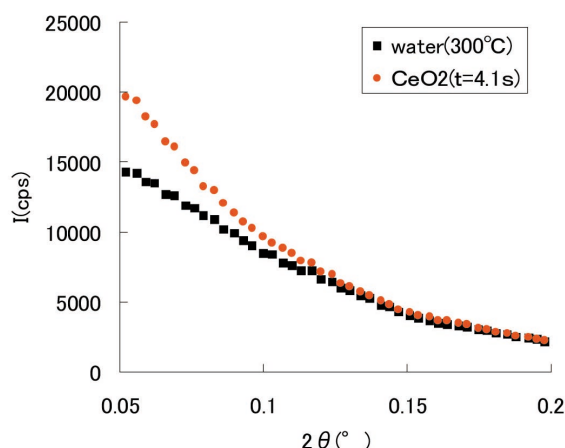
図2 . In-situ SAXS における散乱スペクトル反応温度300℃、圧力30MPa、反応時間4.1秒、原料0.02M 硝酸セリウム水溶液 X線源：MoK、測定時間30min
