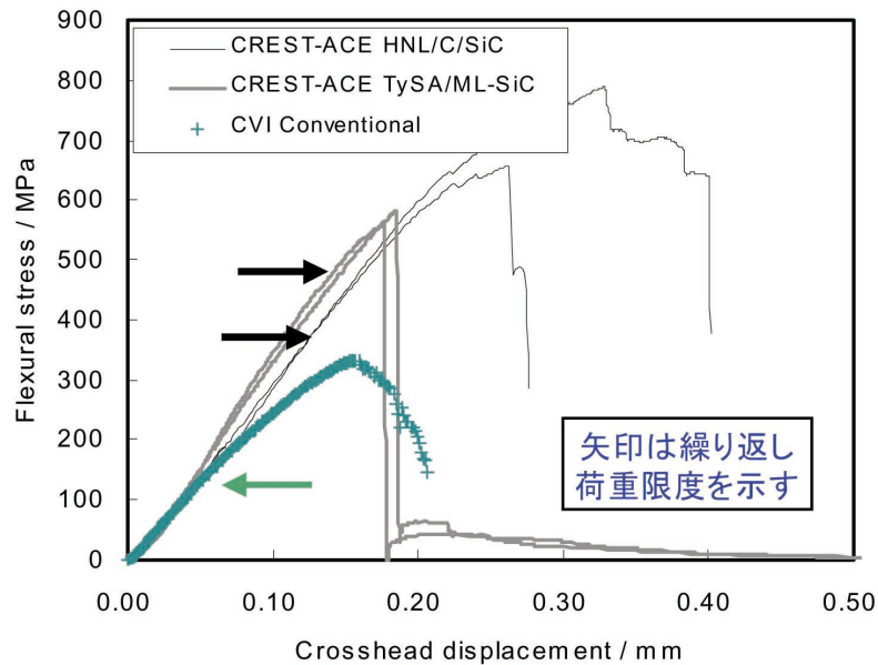
図1 界面制御の高度化によるCVI-SiC/SiCの強度特性改善の例
