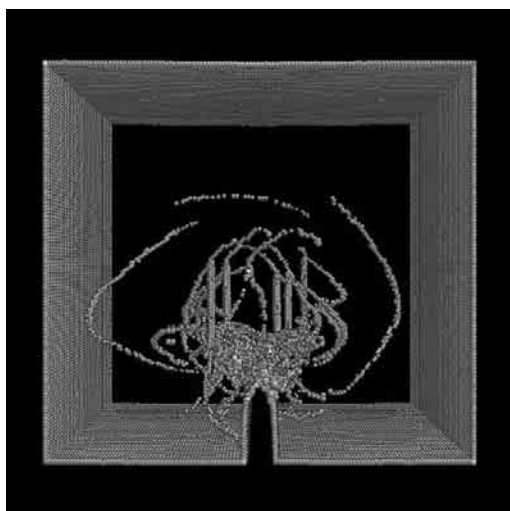
図3 : Cu結晶の破壊過程におけるき裂先端の転位構造 (配位数表示)
