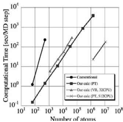
図1：従来法と種々のオーダーN法の計算時間の比較一々の概念図
