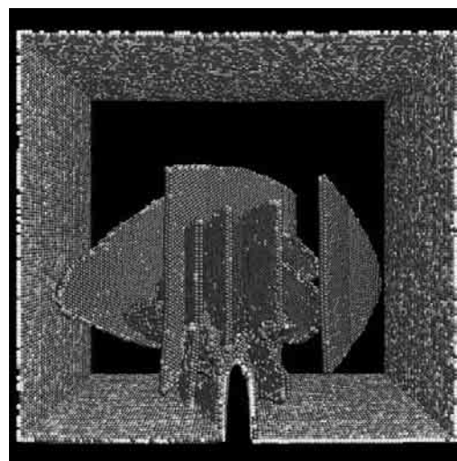
図4 : Cu結晶の破壊過程におけるき裂先端の面欠陥(積層欠陥)構造 (中心対称パラメータ表示)
